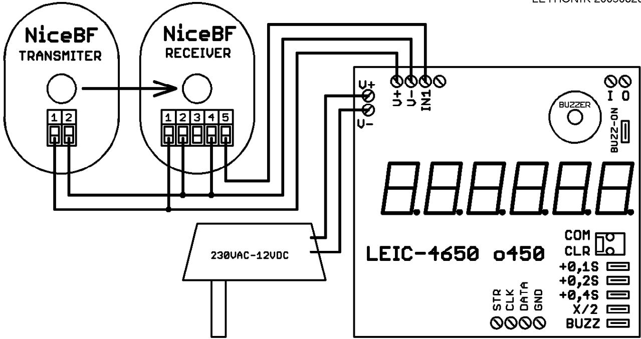
Schemat instalacji o450 - NiceBF
